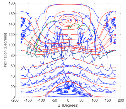
(d) KW4 \phi = 15^\circ , 0.787r_L
